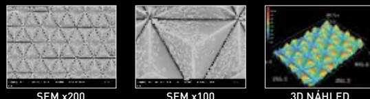
POVRCH KOTOUČE U458
