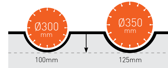
Maks. Kesim Derinliği
