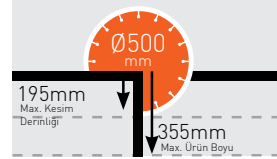
Maksimum Kesim Derinliği
